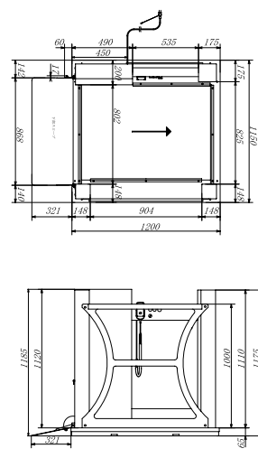
寸法図 直線・左駆動部
