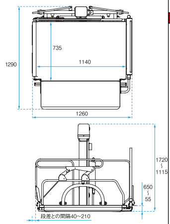
寸法図
