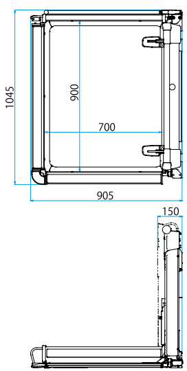
寸法図
